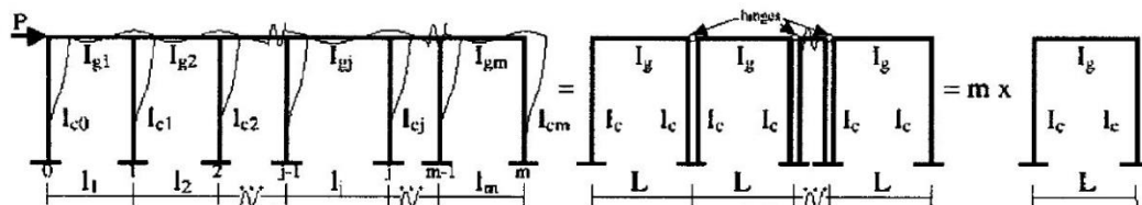
شکل ۱۰- روش پیشنهادی حسینی و ایمان نایینی برای محاسبه سختی طبقات [۲۰]
