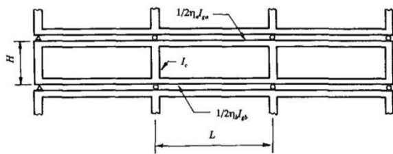
شکل ۸- روش پیشنهادی Schultz برای محاسبه سختی [۱۷]
