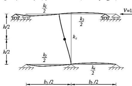
شکل ۹- روش پیشنهادی Paulay and Priestley برای محاسبه سختی [۱۹]
