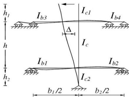
شکل ۱۲- روش پیشنهادی Caterino, Cosenza and Azmoodeh
