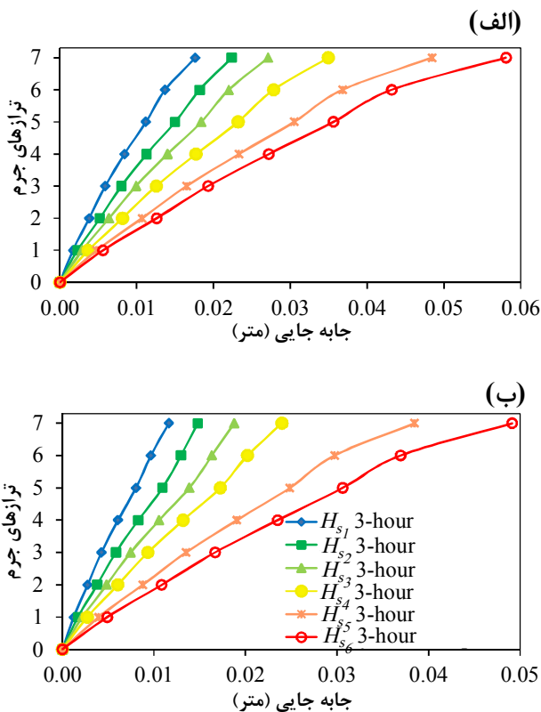
شکل ۱۰- احتمال فزون‌ی ۵۰٪ برای بیشینه جابه‌جایی عرشه در تمامی ترازهای جرمی برای سری‌های زمانی (الف) رکوردهای امواج تصادفی ۳ ساعته و (ب) موج نو افزایشی اصلاح شده
