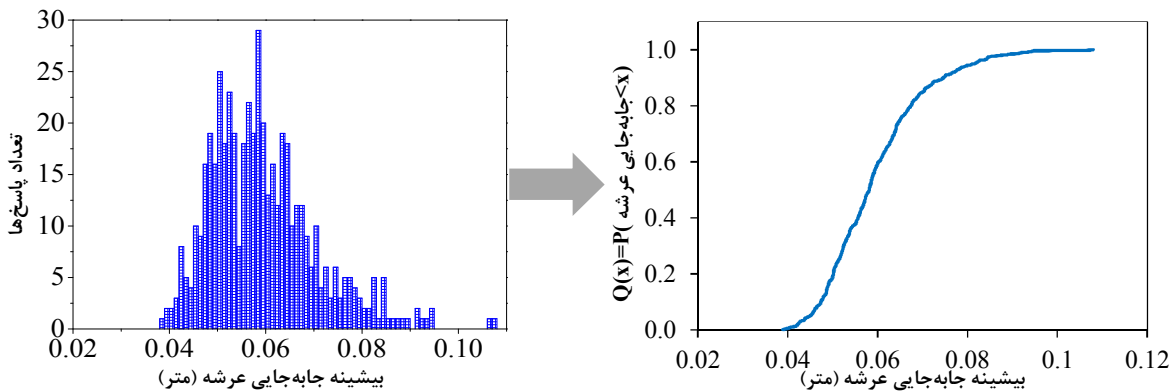
شکل ۷ - جابه‌جایی‌های حدی عرشه و توزیع تجمعی آن برای رکوردهای امواج تصادفی ۳ ساعته
