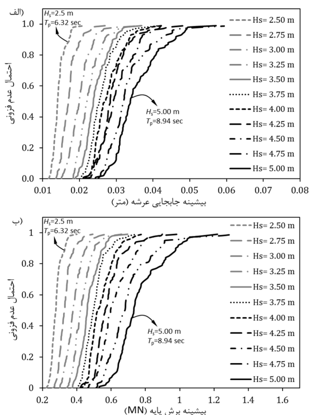
شکل ۷- توزیع احتمال تجمعی تحلیل‌های سه ساعته. الف) جابجایی بیشینه عرشه، ب) بیشینه برش پایه
