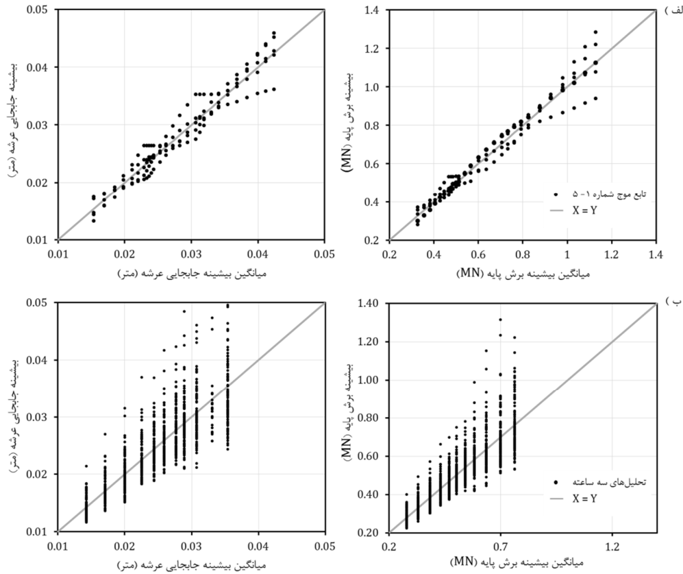
شکل ۱۰ - آزمایش فرضی سکوه‌های دریایی به روش زمان دوام موج
